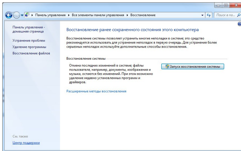
Рис.203.ДиалоговоеокноВосстановление
