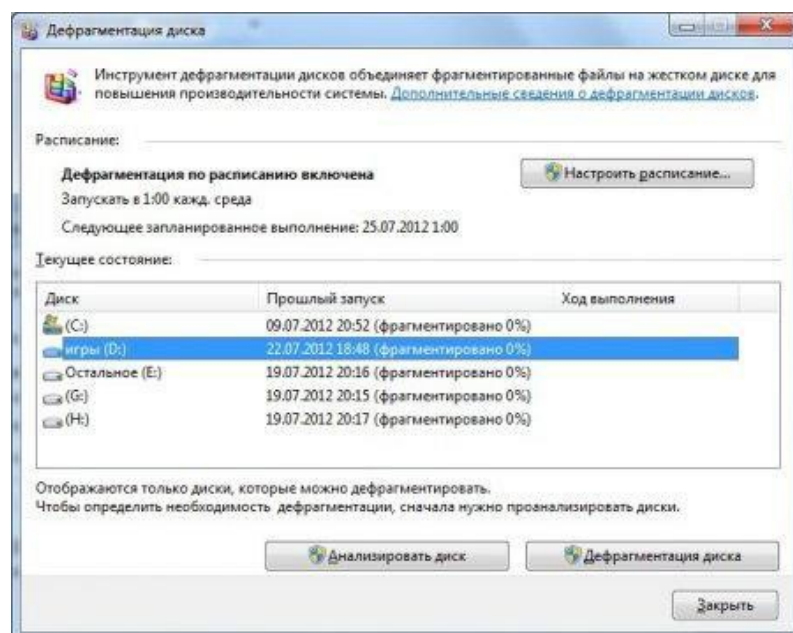
Рис.39.Результатанализадиска
