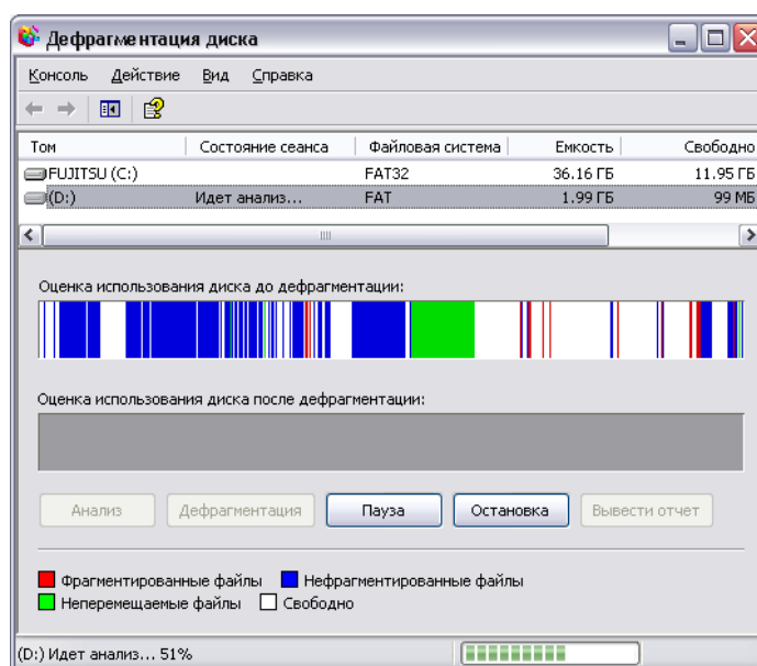
Рис.34.ДиалоговоеокноДефрагментациядиска
