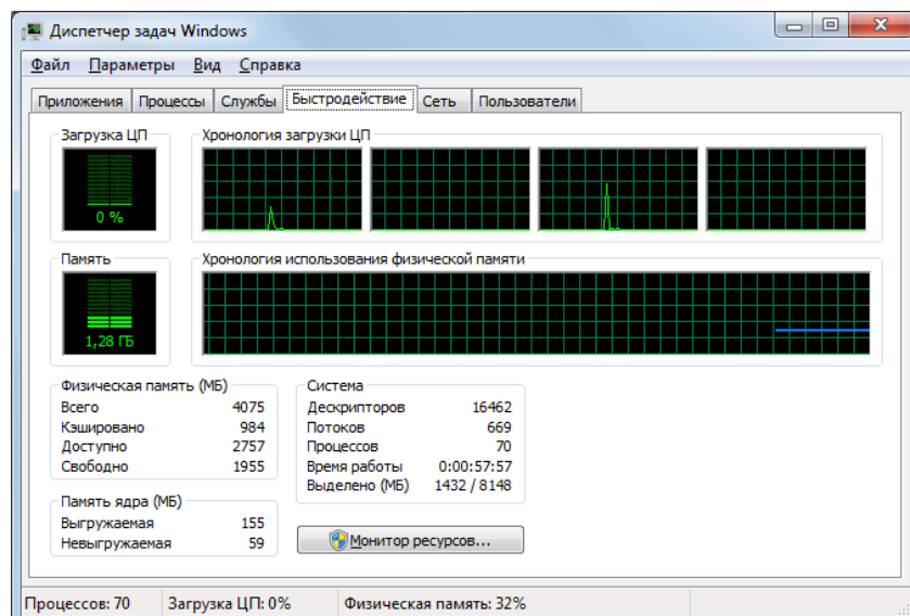
Рис.79.Вкладка Быстродействие
