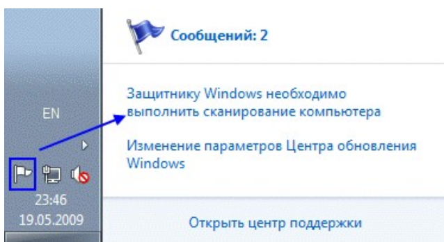
Рис.189.Областьуведомлений
