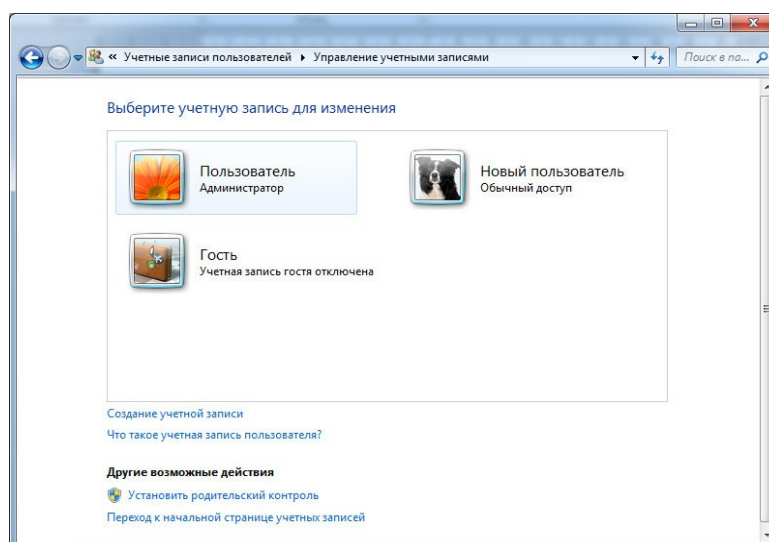
Рис.135.СозданаучетнаязаписьНовыйпользователь
