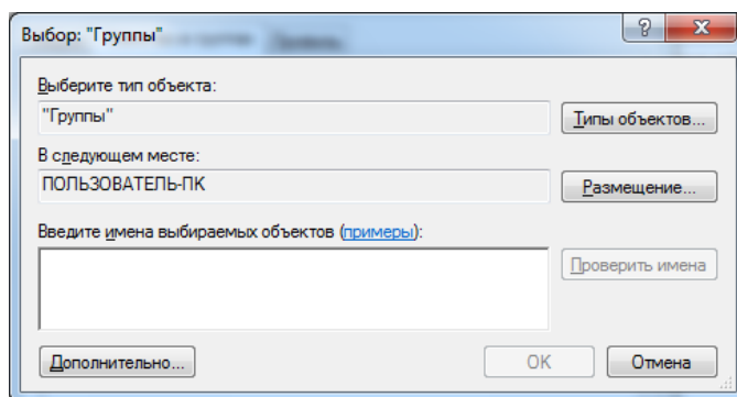
Рис.150.ОкноВыбор:Группы
