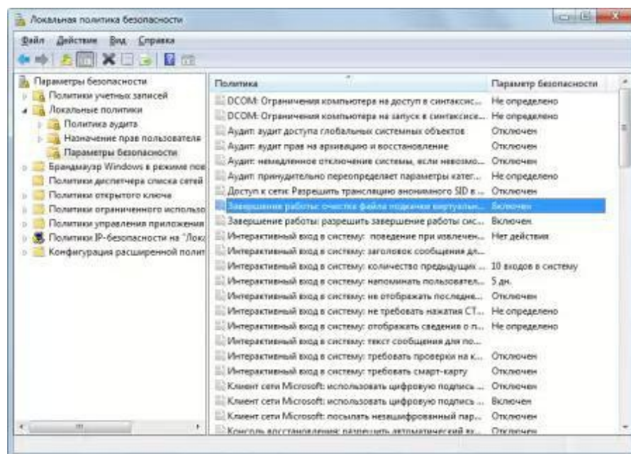
Рис.86.ДиалоговоеокноЛокальнаяполитикабезопасности
