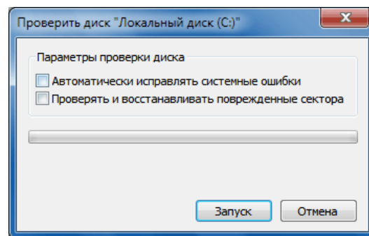
Рис.32.Параметры проверки
