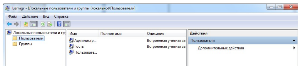
Рис.144.ДиалоговоеокноЛокальныепользователиигруппы
