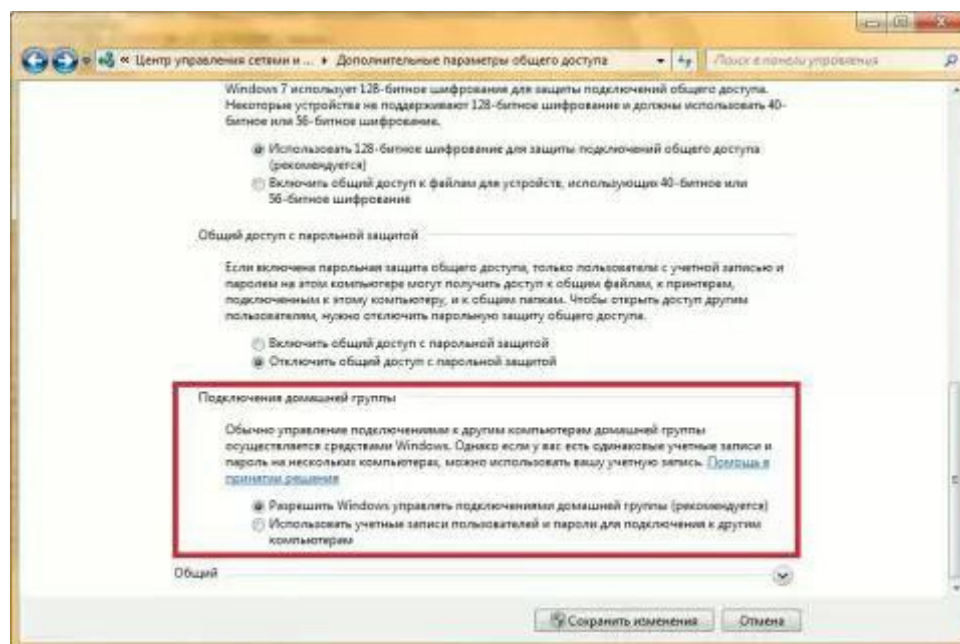
Рис.185.Настройкаподключениядомашнейгруппы
