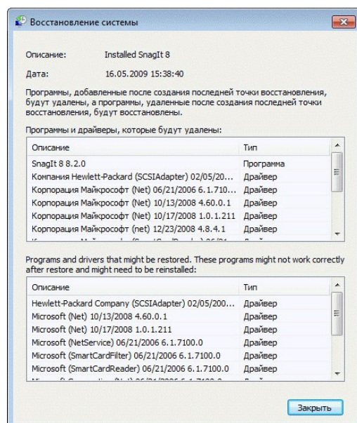
Рис.211.Список программ
