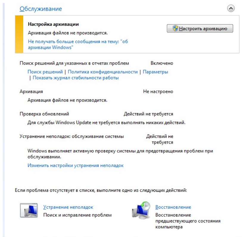
Рис. 192. Раздел Обслуживание
