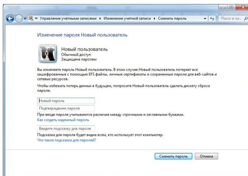
Рис.138.ИзменениепаролядляучетнойзаписиНовыйпользователь
