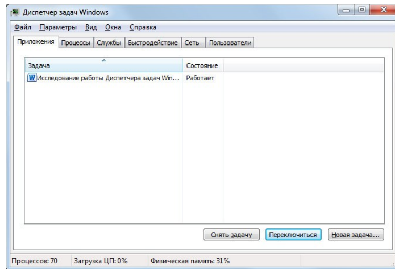
Рис.76. Вкладка Приложения
