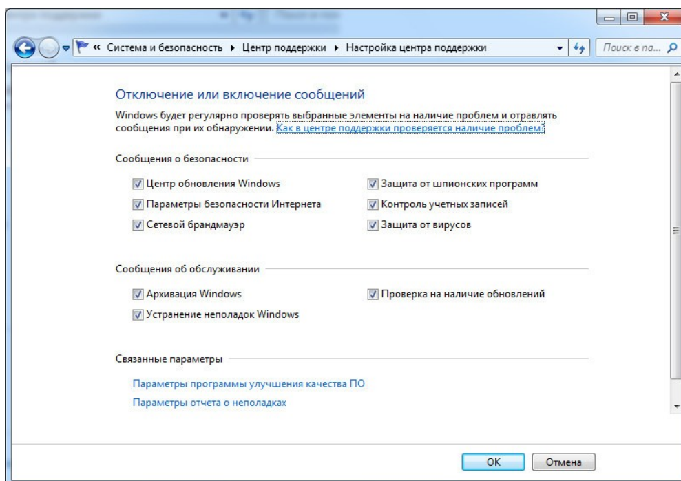
Рис.193.Параметрынастройки
