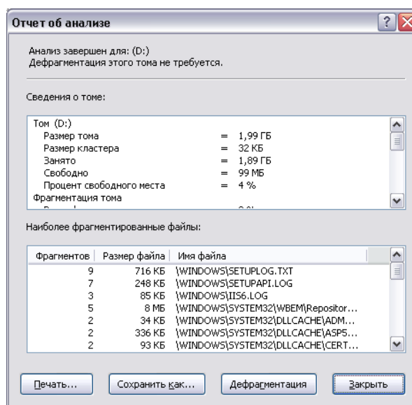
Рис.35.ОтчетобанализедискаD:
