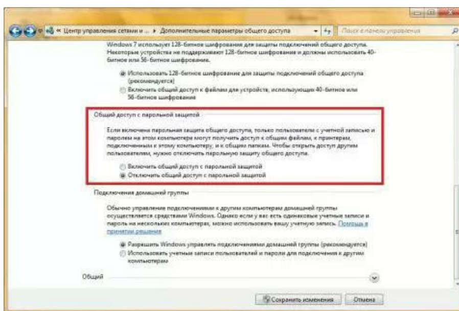
Рис.184.Отключениепарольнойзащитыдляобщегодоступакфайлами папкам
