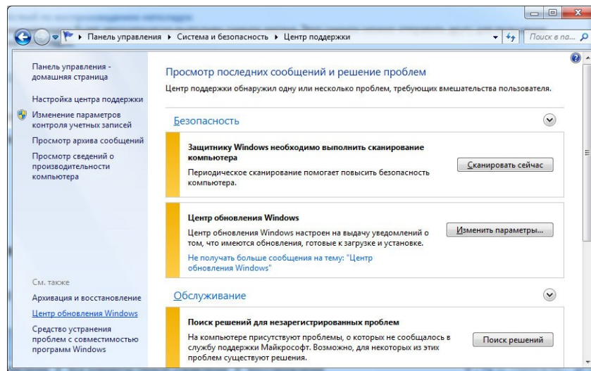
Рис.201.ДиалоговоеокноЦентрподдержки
