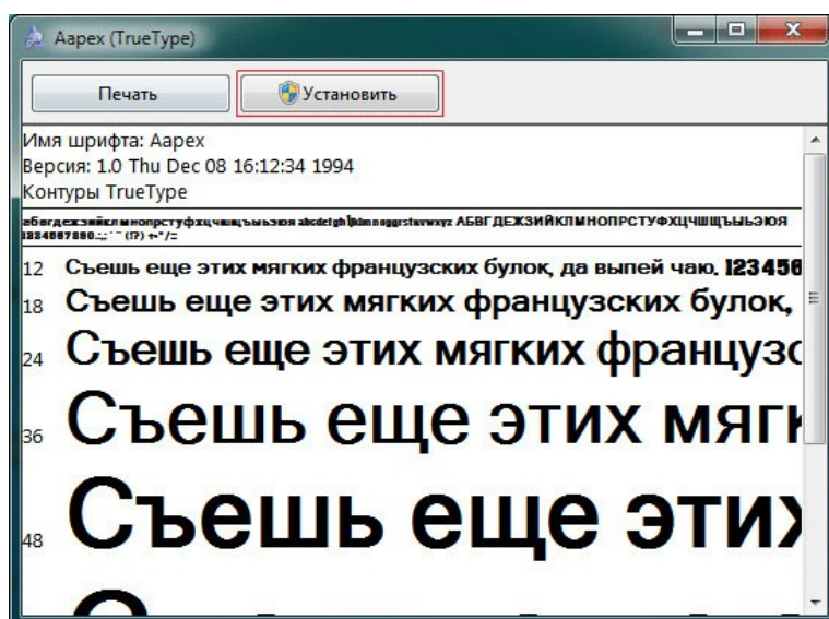
Рис.29.ШрифтАарех
