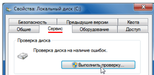
Рис.31.Вкладка Сервис
