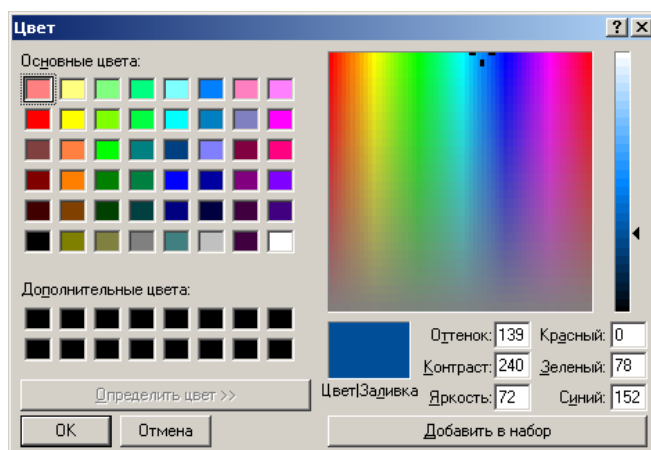
Рис.15.ДиалоговоеокноЦвет
