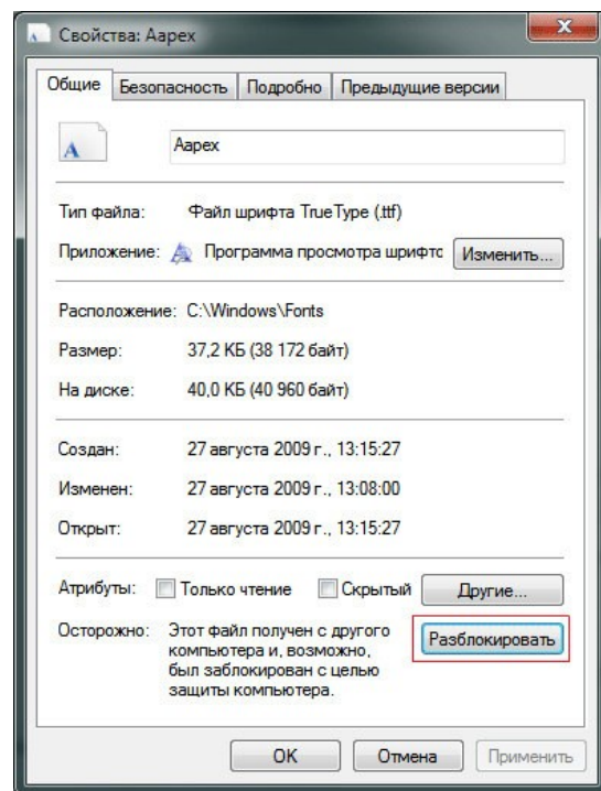
Рис.28. Свойства шрифта
