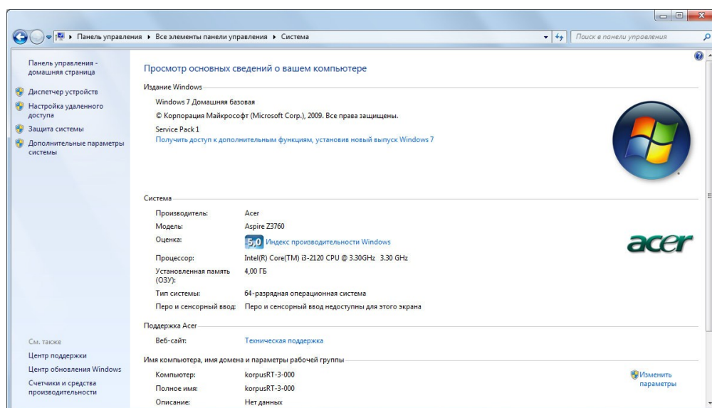
Рис.82.Панельуправления.Система
