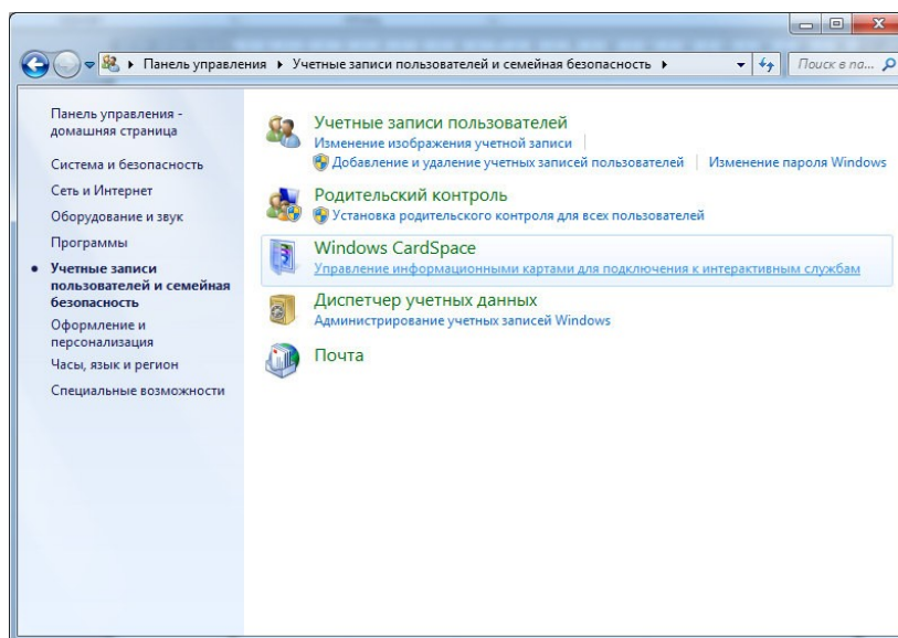
Рис.131.Панельуправления.Учетныезаписипользователей
