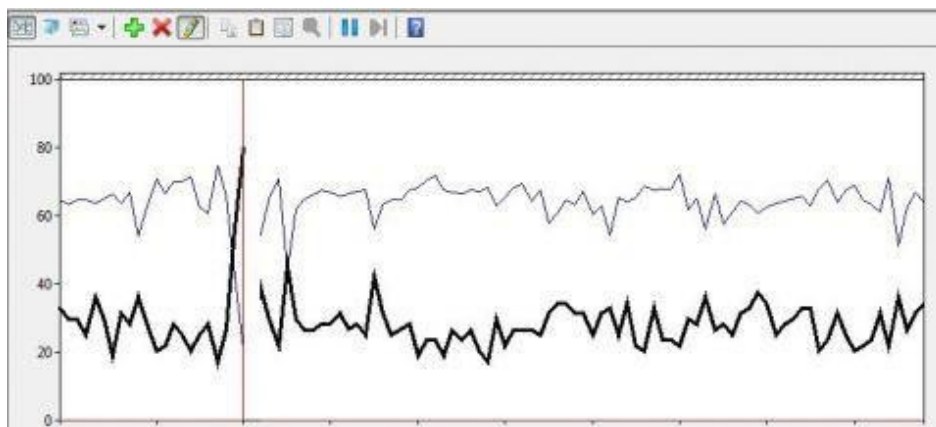
Рис.105.Выделенныйсчетчикпроизводительности
