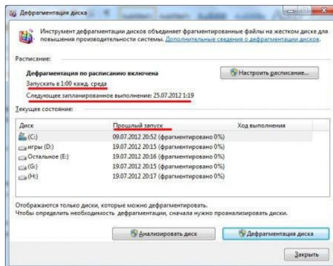
Рис.36.ДиалоговоеокноДефрагментациядиска
