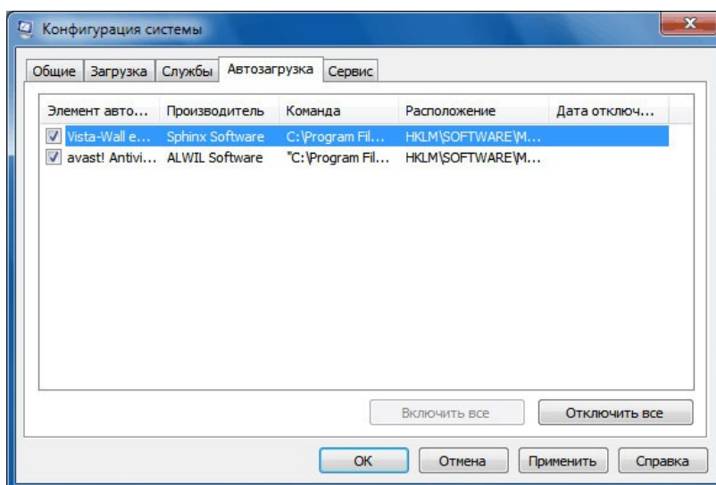
Рис.74 Вкладка Автозагрузка
