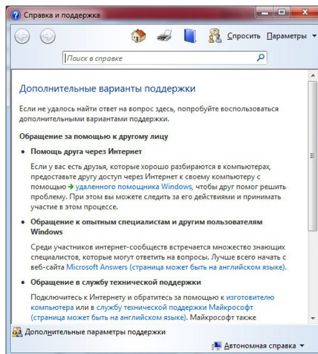
Рис.202.ДиалоговоеокноСправкаиподдержка
