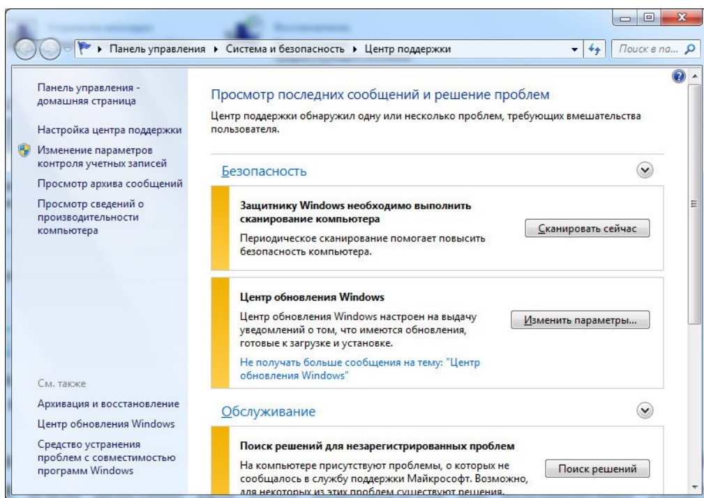
Рис.187.ДиалоговоеокноЦентрподдержки
