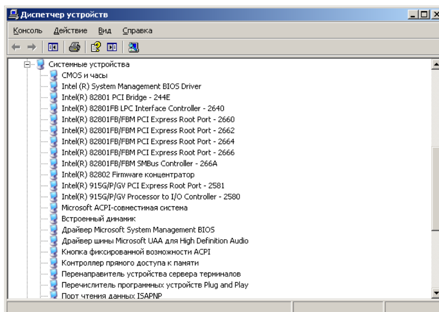
Рис.94.ДиалоговоеокноДиспетчерустройств
