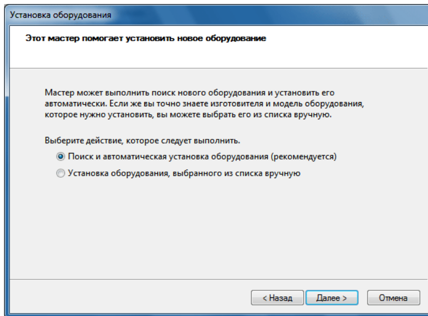
Рис.126. Установка оборудования
