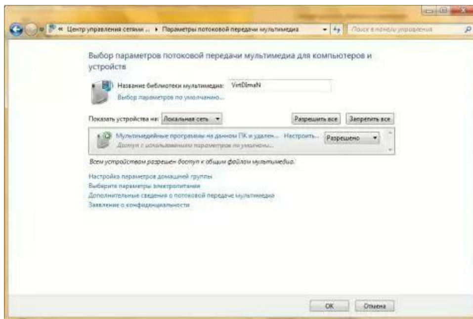
Рис.183.Параметрыпотоковойпередачимультимедиа
