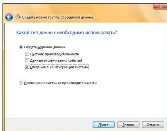
Рис.113.Выбортипаданныхдлягруппысборщиковданных
