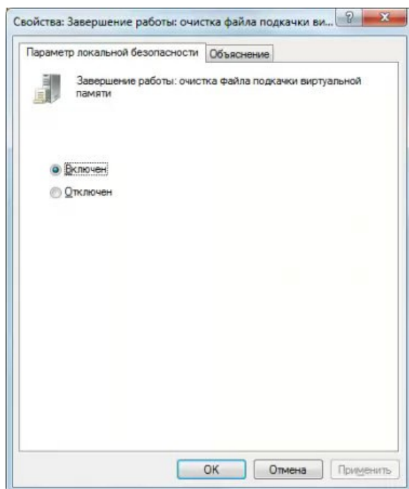
Рис.87.ВкладкаПараметрлокальной безопасности
