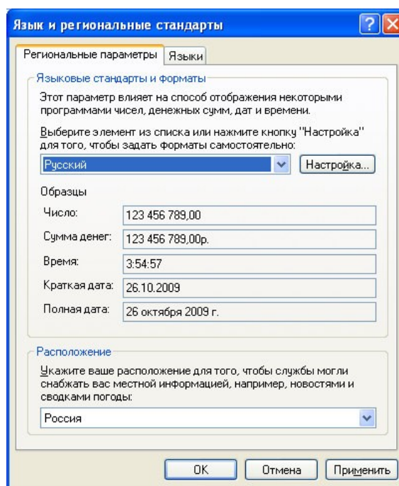
Рис.7.Языкиирегиональныестандар- ты
