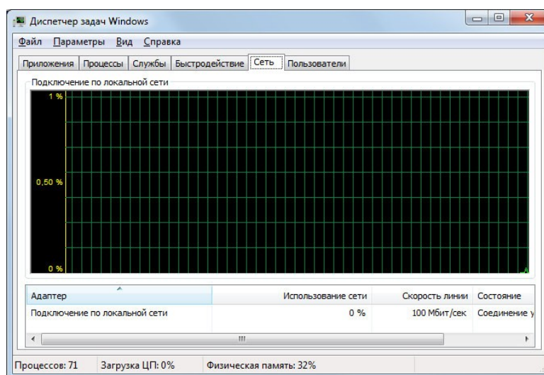
Рис.80.Вкладка Сеть
