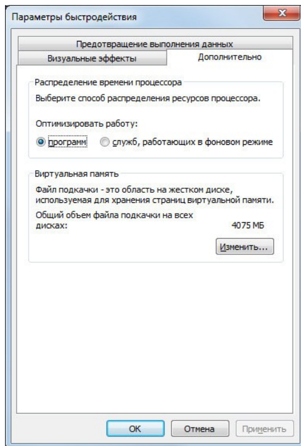
Рис.84.Параметрыбыстродей- ствия
