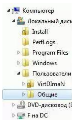
Рис.175.Папка Общие
