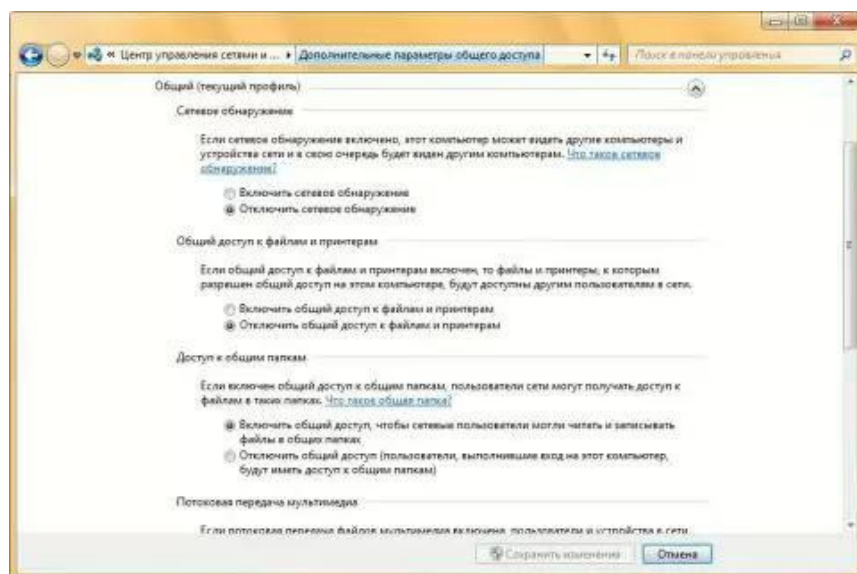
Рис.172.ОкноДополнительныепараметрыобщегодоступа
