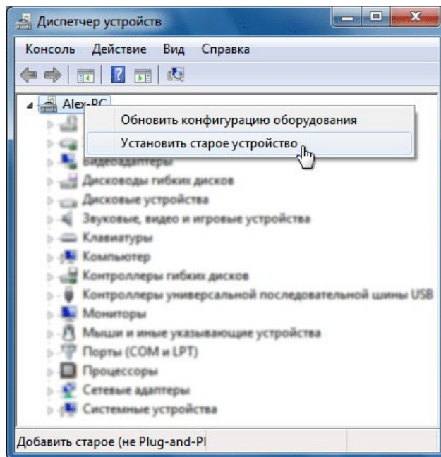
Рис.124.ОкноДиспетчерустройств
